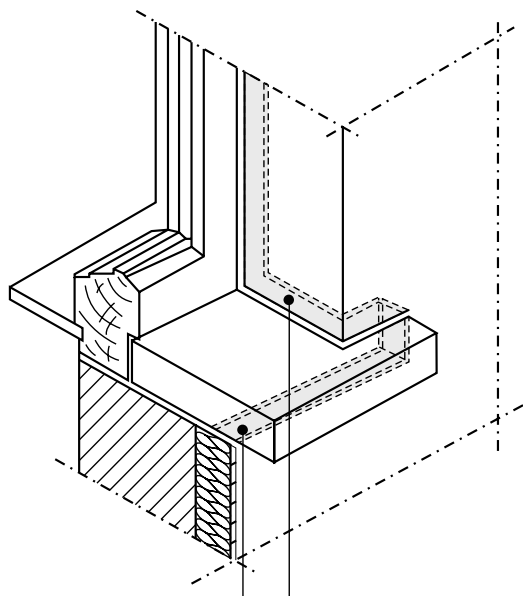
Tesniaca páska (trvalo pružný tmel)
